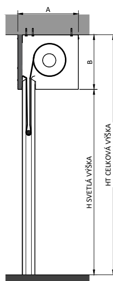
REZ UPEVNENIE DO OTVORU
