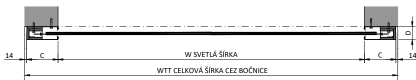
PÔDORYS - UPEVNENIE NA OTVOR
