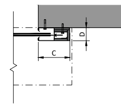
DETAIL UPEVNENIA VODIACICH LÍŠŤ DO OTVORU
