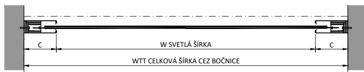
PÔDORYS - UPEVNENIE DO OTVORU
