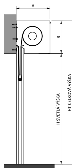
REZ UPEVNENIE NA OTVOR
