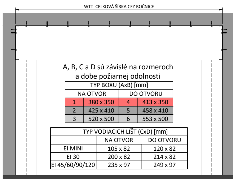
POHĽAD - UPEVNENIE DO OTVORU
