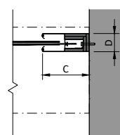
DETAIL UPEVNENIA VODIACICH LÍŠŤ DO OTVORU
